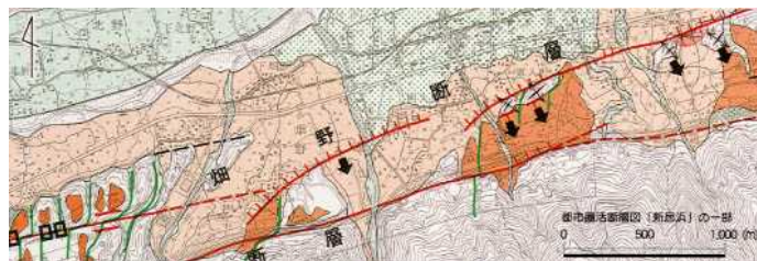
都市圏活断層図のサンプル(一部)
